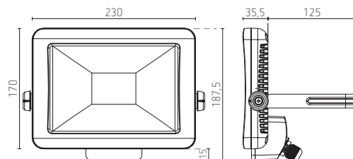
theLeda B30L
