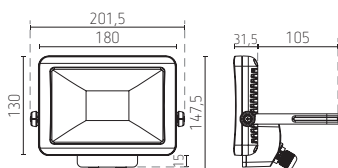
theLeda B10L
