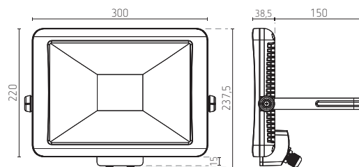
theLeda B50L
